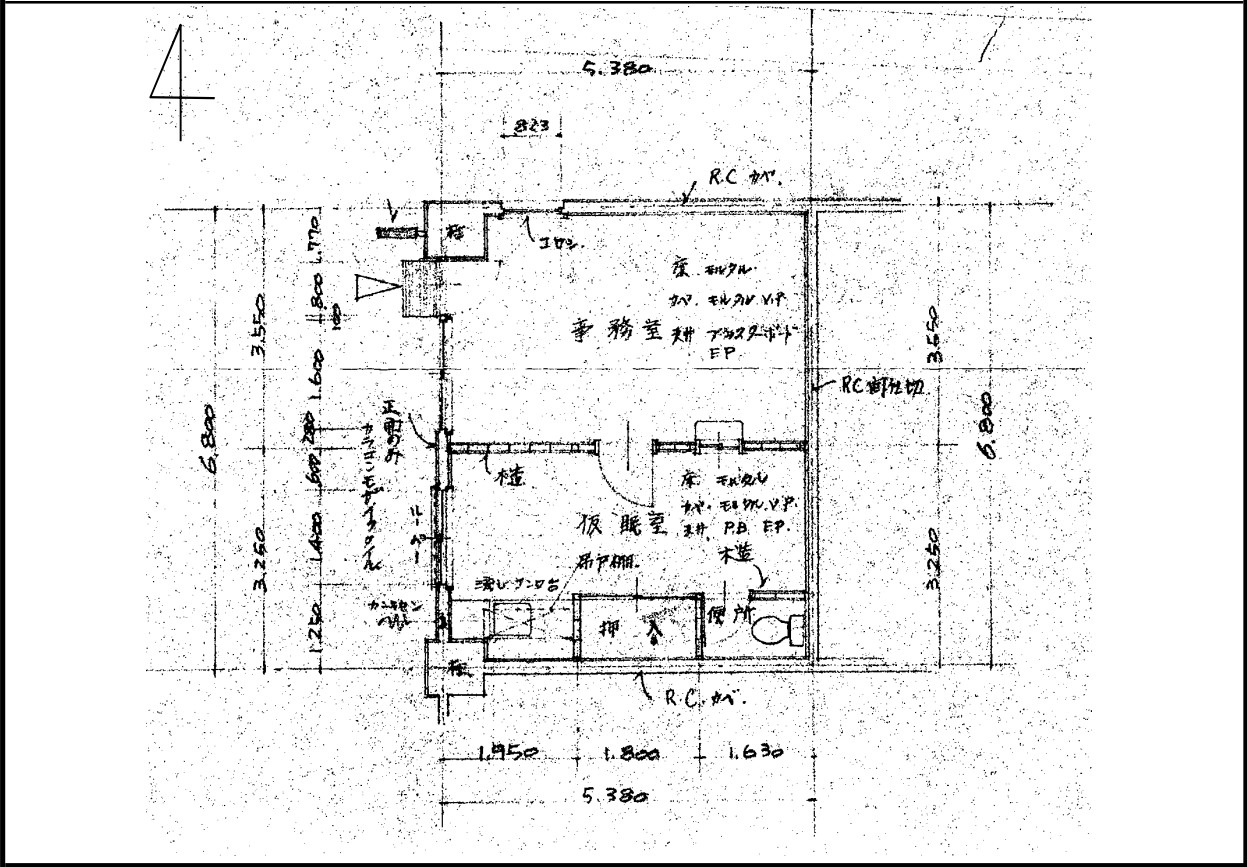
平面図（事務所部分）
